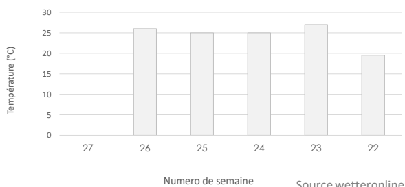
Evolution des températures (moyenne France)
