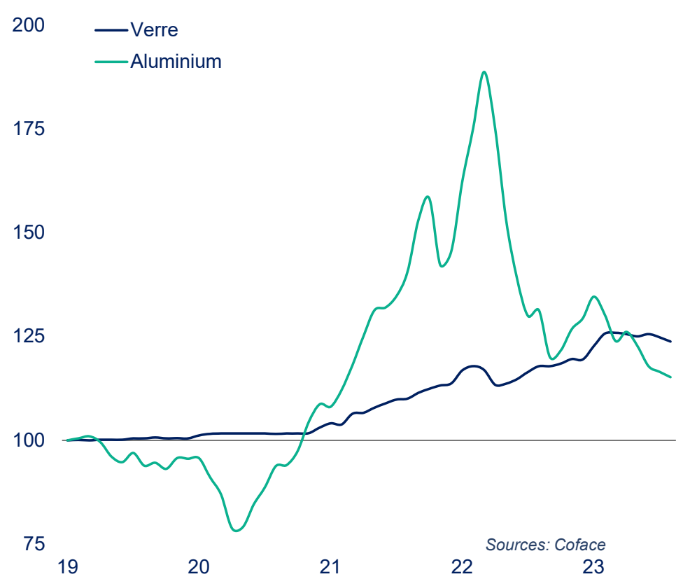
Coûts des intrants packaging – France (IPP index, 2019=100)
